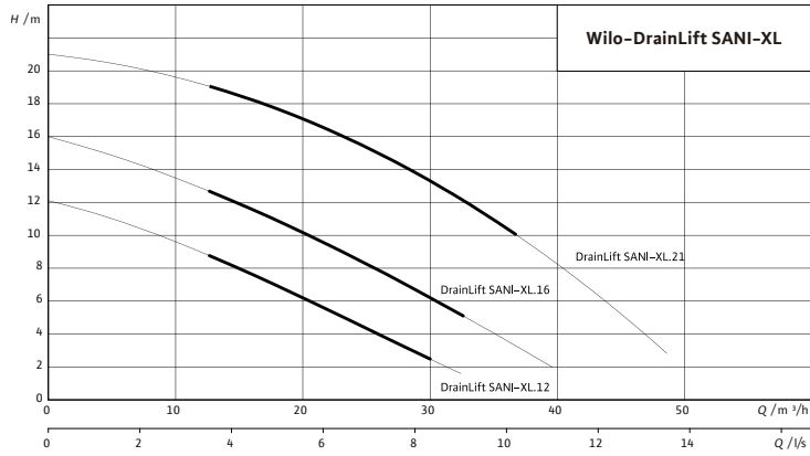
特性曲线图
