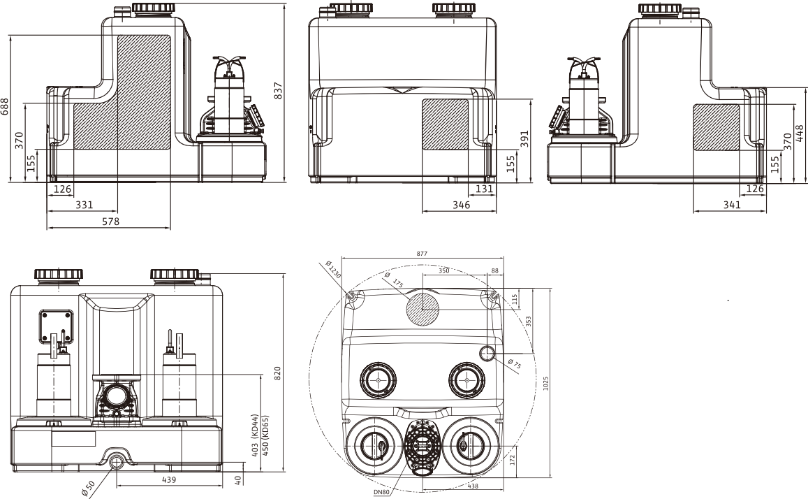
尺寸图
