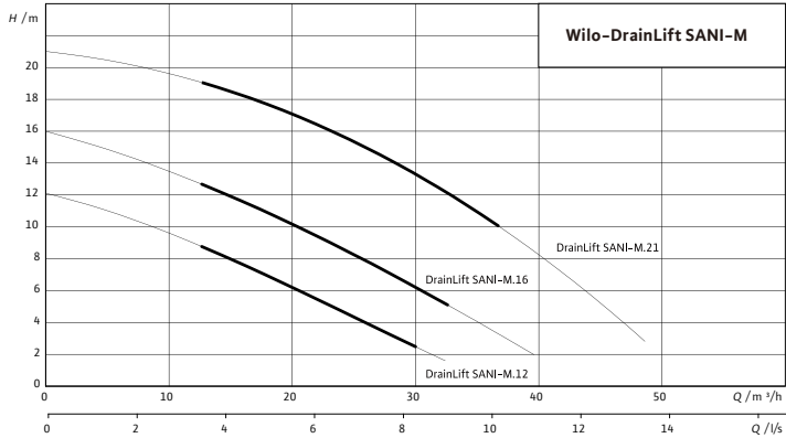
特性曲线图
