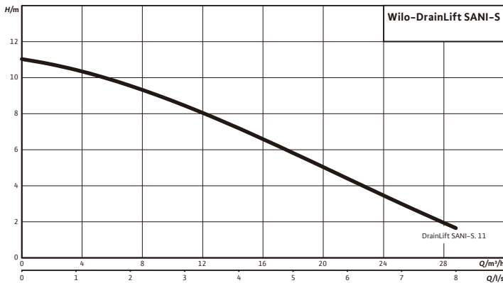
特性曲线图
