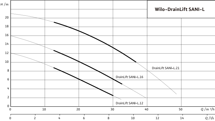
特性曲线图
