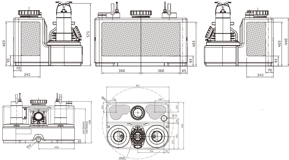
尺寸图
