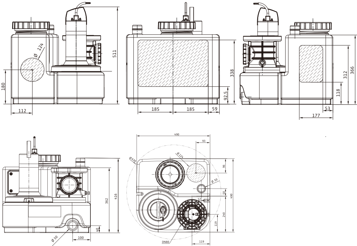
尺寸图
