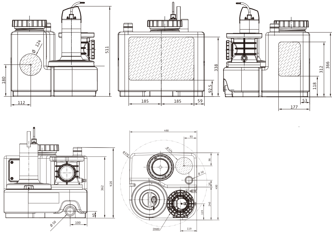
尺寸图
