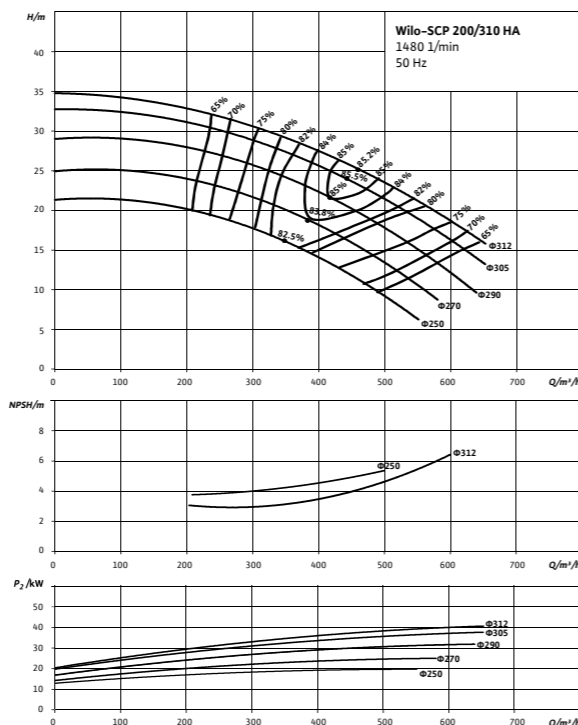
Wilo-SCP 200/310 HA
