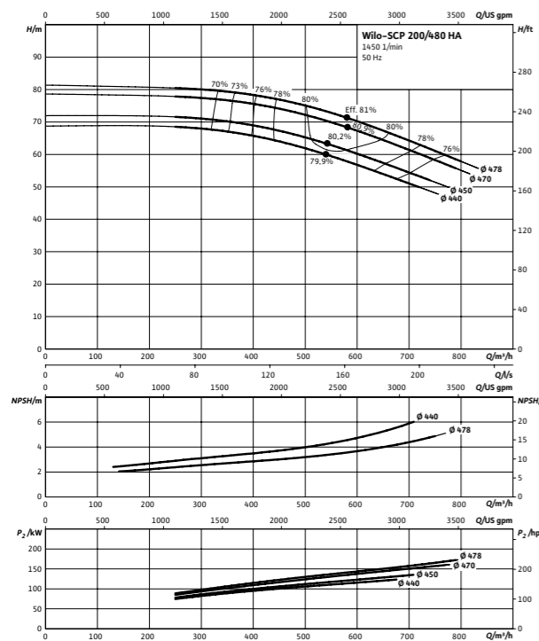
Wilo-SCP 200/480 HA
