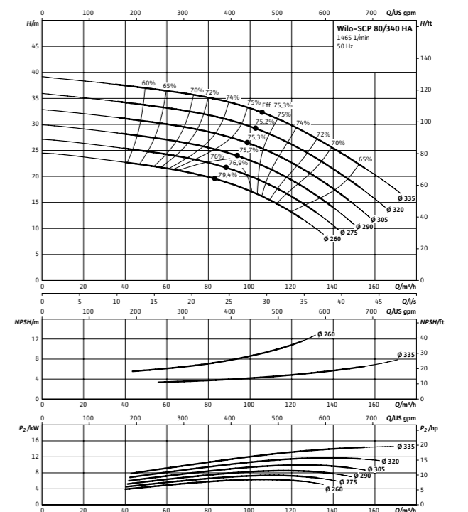
Wilo-SCP 80/340 HA
