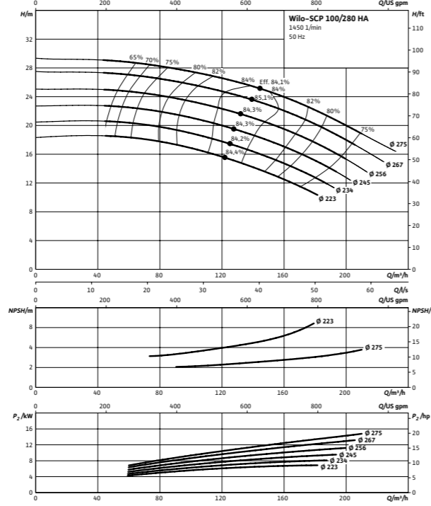
Wilo-SCP 100/280 HA
