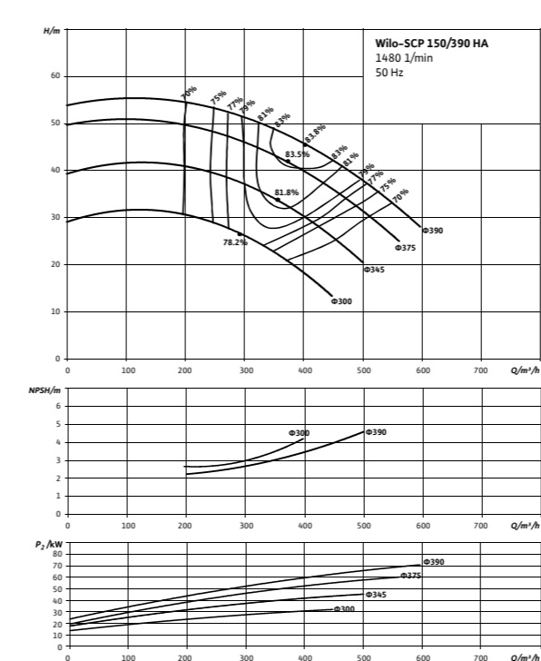
Wilo-SCP 150/390 HA
