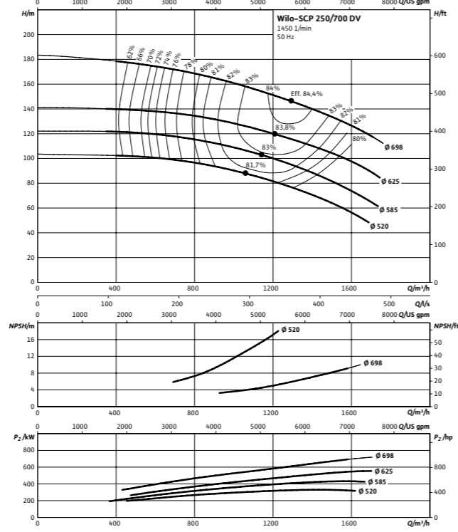
Wilo-SCP 250/700 DV
