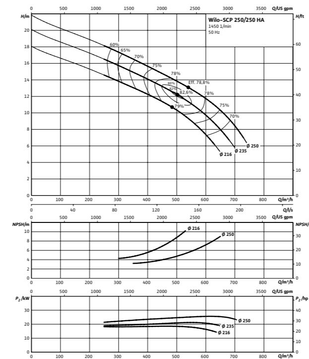
Wilo-SCP 250/250 HA
