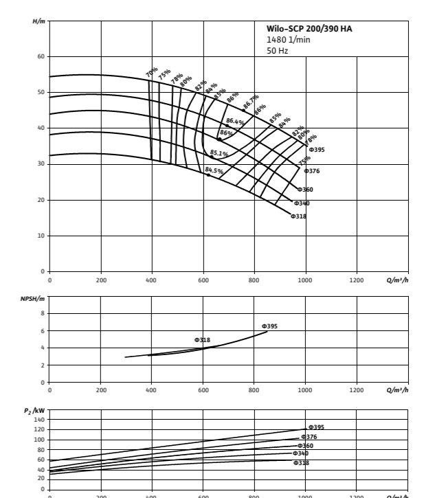
Wilo-SCP 200/390 HA
