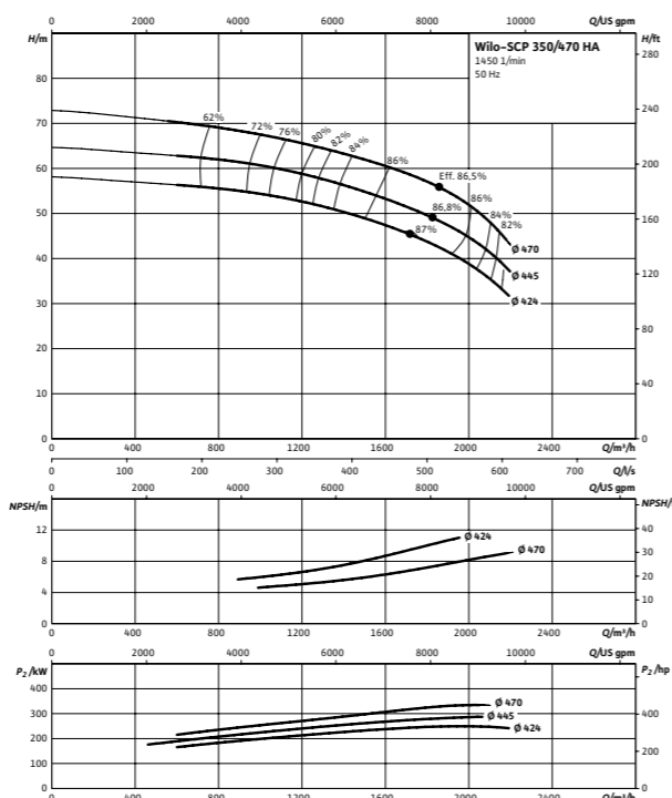
Wilo-SCP 350/470 HA
