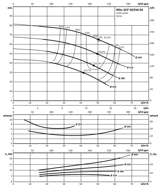
Wilo-SCP 50/340 DS
