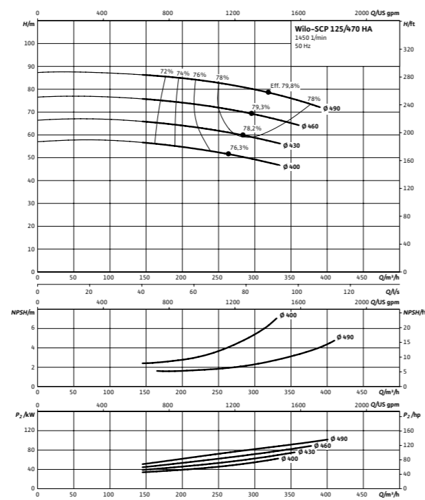
Wilo-SCP 125/470 HA
