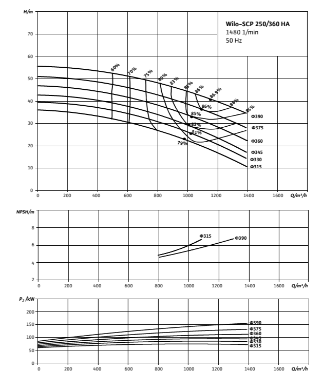
Wilo-SCP 250/360 HA
