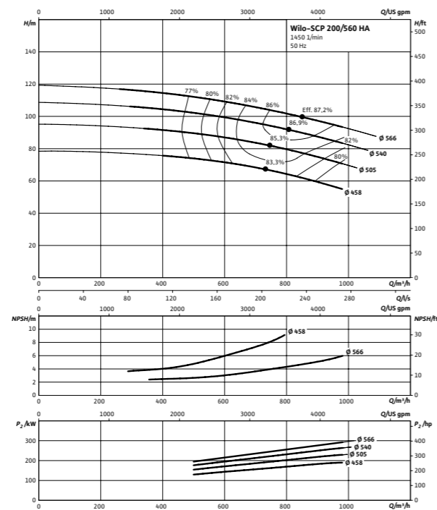
Wilo-SCP 200/560 HA
