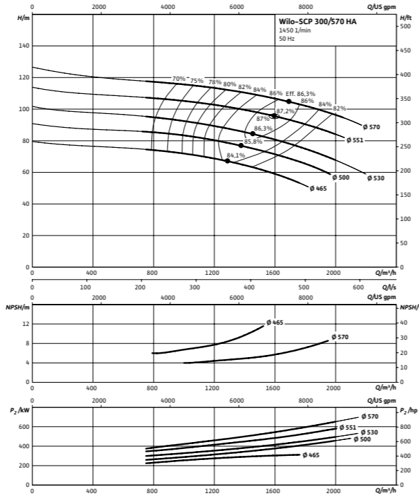
Wilo-SCP 300/570 HA
