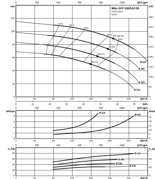
Wilo-SCP 100/410 DS
