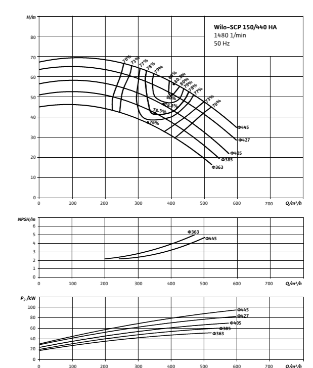
Wilo-SCP 150/440 HA
