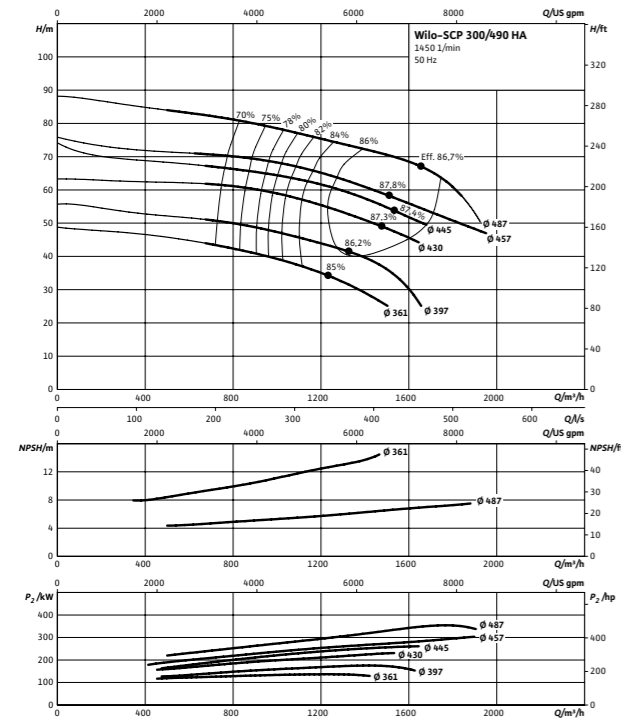
Wilo-SCP 300/490 HA
