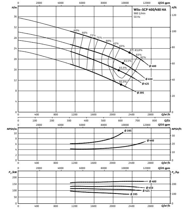
Wilo-SCP 400/480 HA
