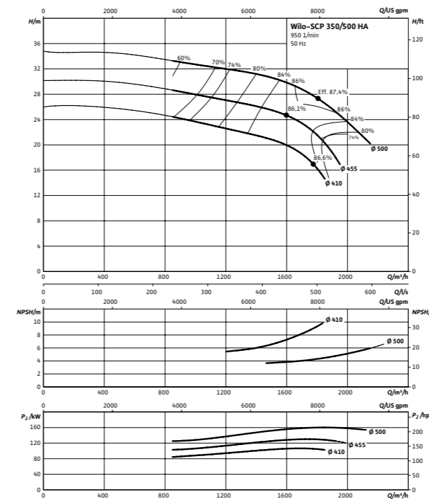
Wilo-SCP 350/500 HA
