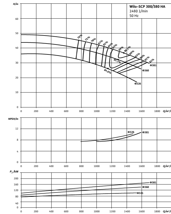
Wilo-SCP 300/380 HA
