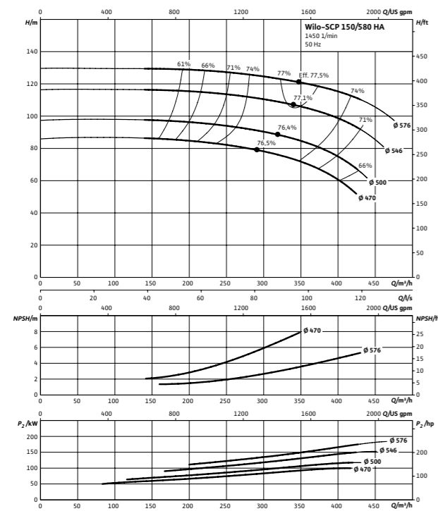
Wilo-SCP 150/580 HA
