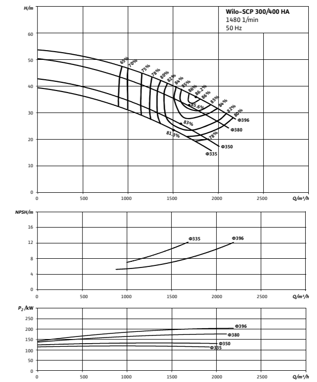
Wilo-SCP 300/400 HA
