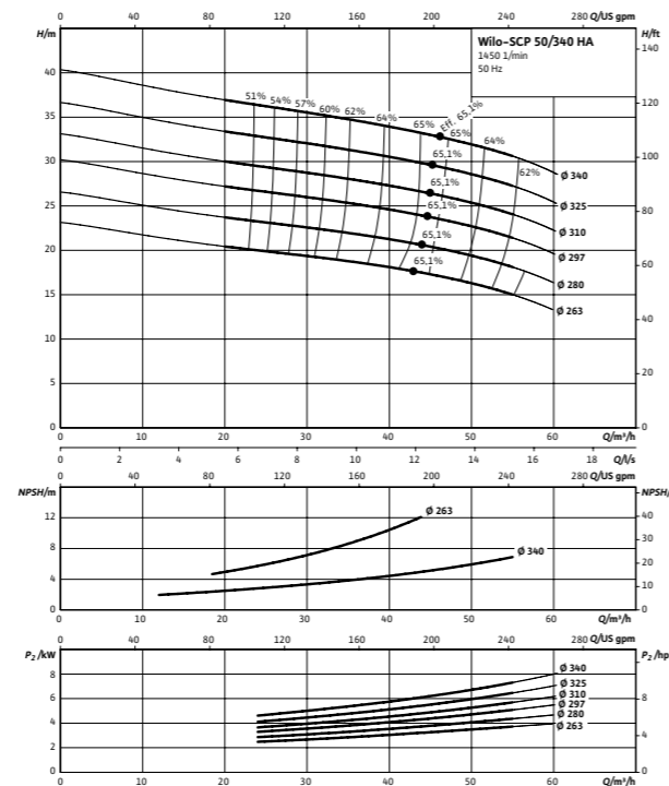
Wilo-SCP 50/340 HA
