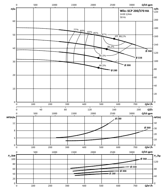
Wilo-SCP 200/370 HA
