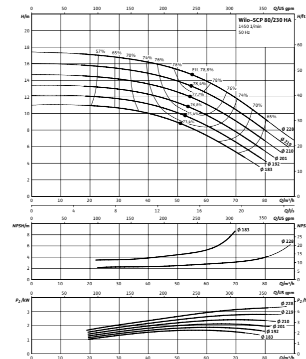
Wilo-SCP 80/230 HA
