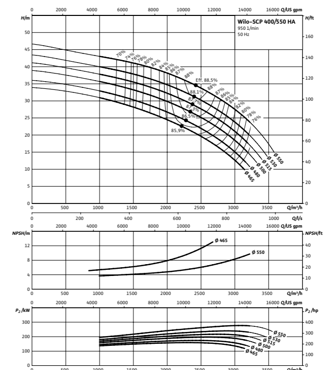
Wilo-SCP 400/550 HA
