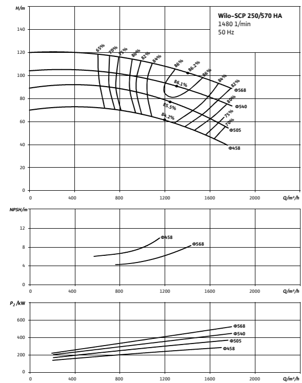
Wilo-SCP 250/570 HA
