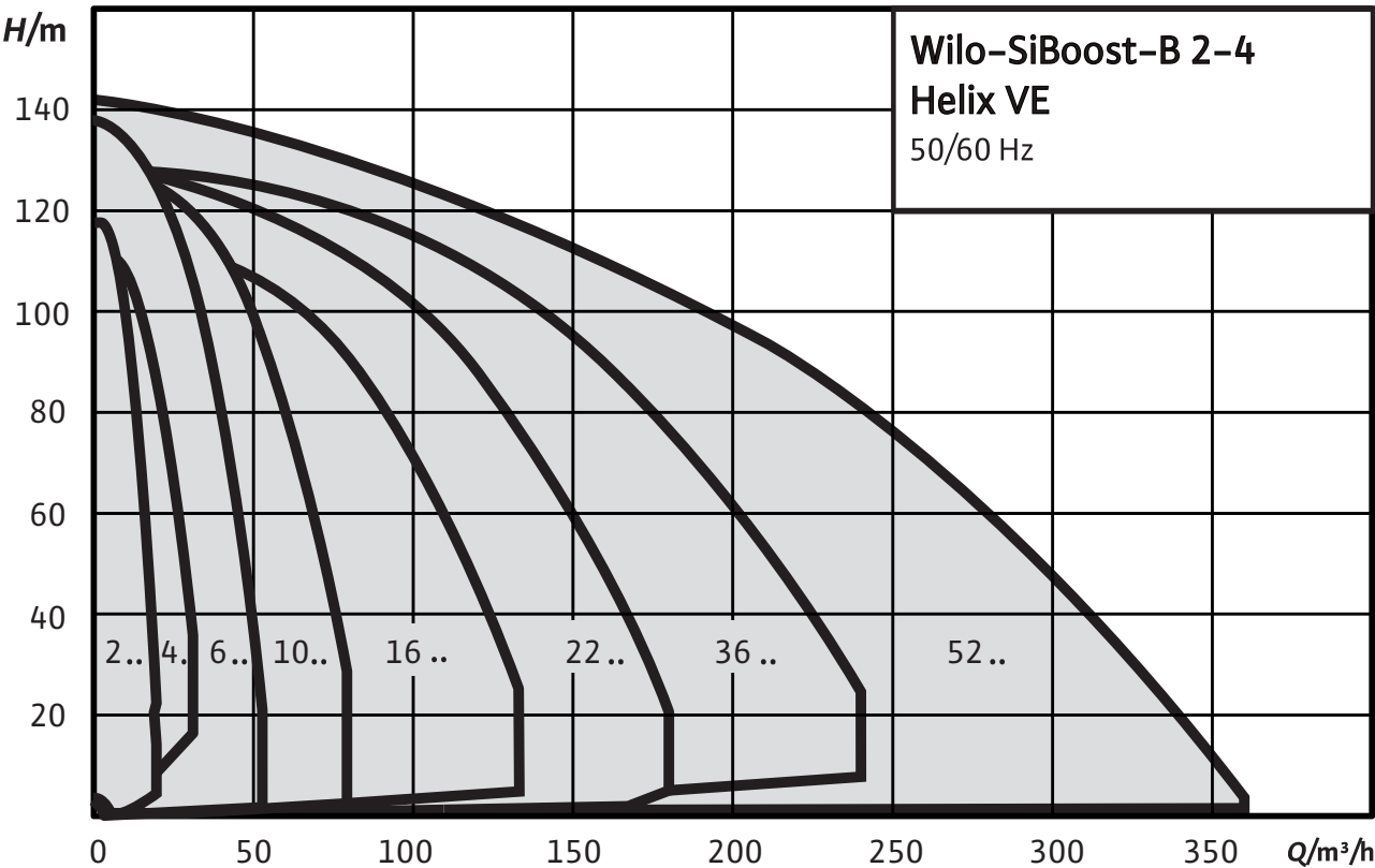
Wilo-SiBoost B 2-4 Helix VE 型谱图
