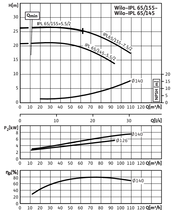
Wilo-IPL 65/145-5.5/2 - 65/155-7.5/2
