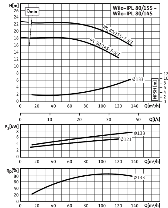
Wilo-IPL 80/145-5.5/2 - 80/155-7.5/2
