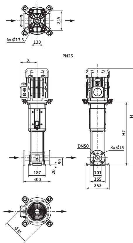
尺寸图 Helix V 16, PN 25
