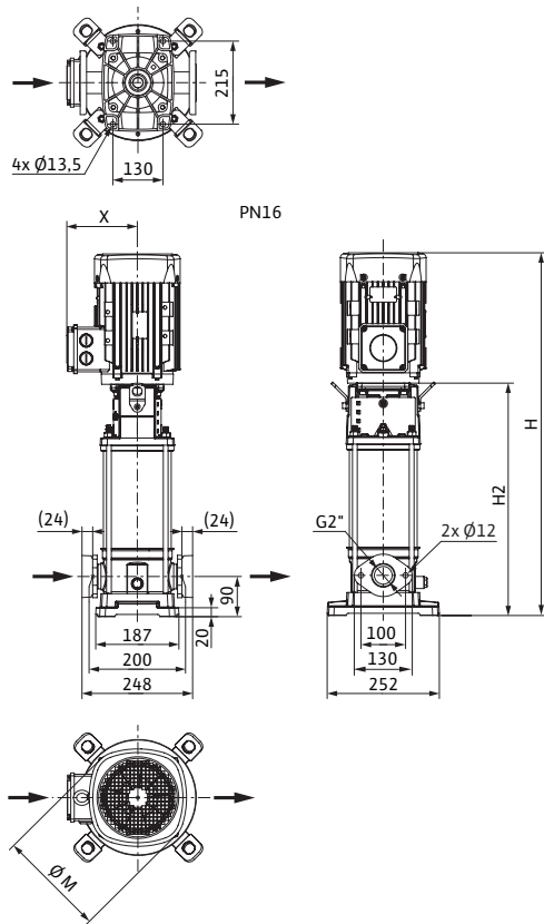
尺寸图 Helix V 16, PN 16
