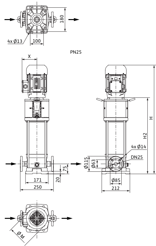
尺寸图 Helix V 2/V 4, PN 25
