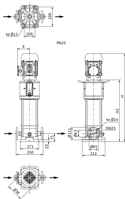
尺寸图 Helix V 2/V 4, PN 25
