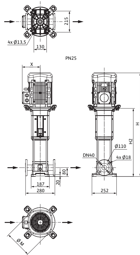
尺寸图 Helix V 10, PN 25
