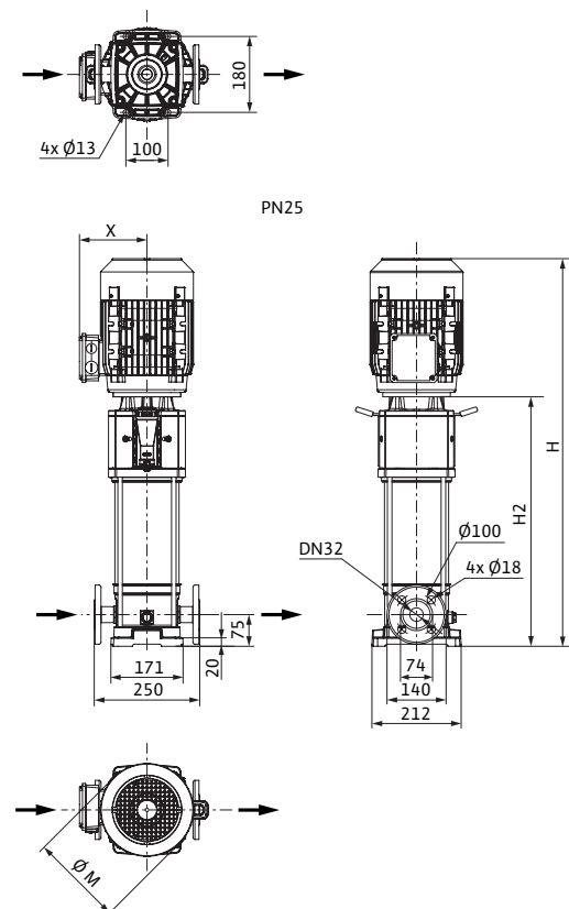
尺寸图 Helix V 6, PN 25
